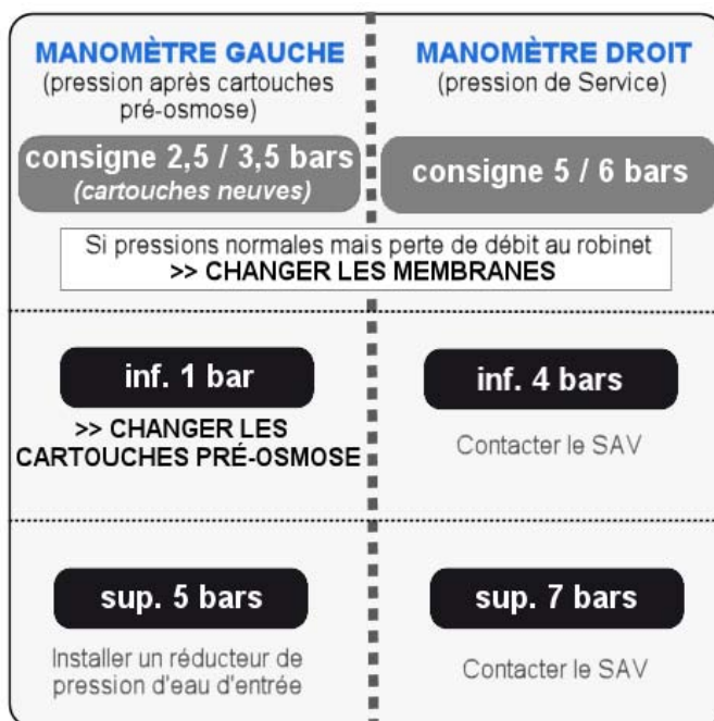
(Récapitulatif des pressions fonctionnelles de l'osmoseur RO ust -3000)
